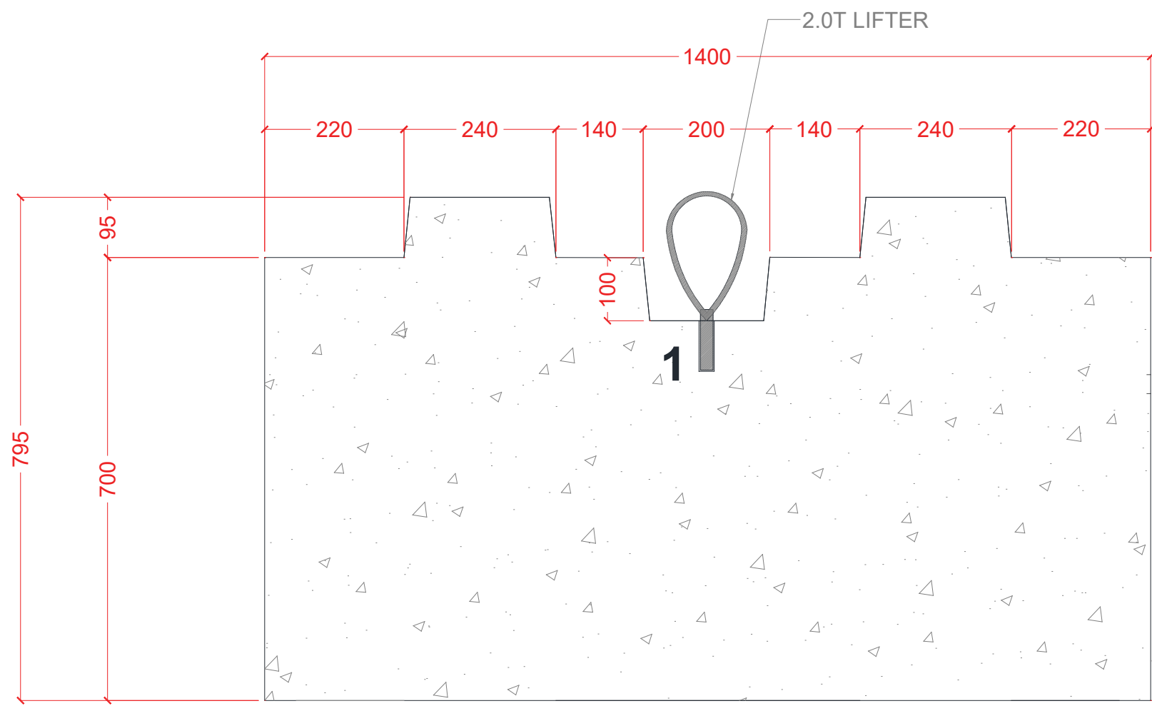
SECTION A-A
