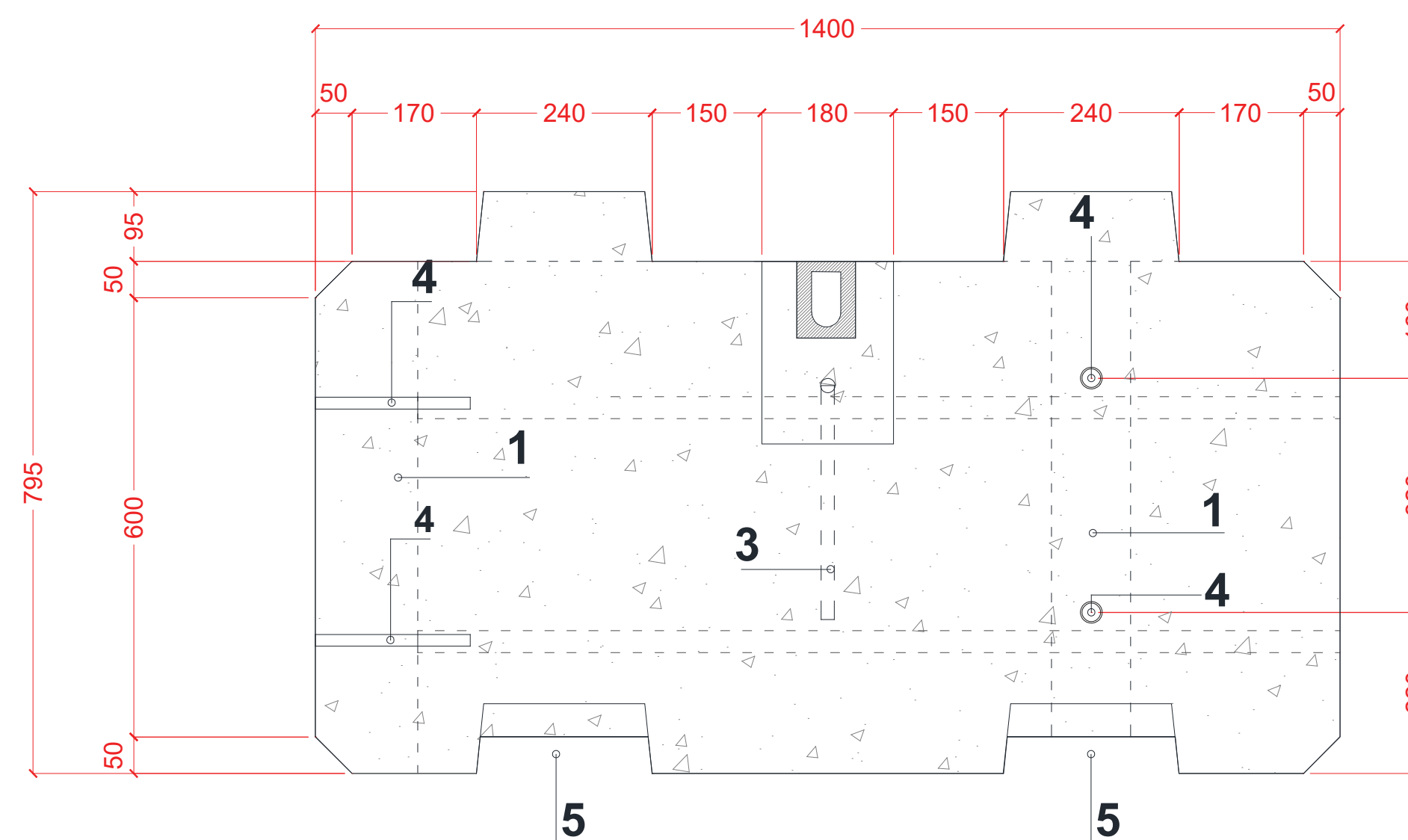
SECTION A-A
